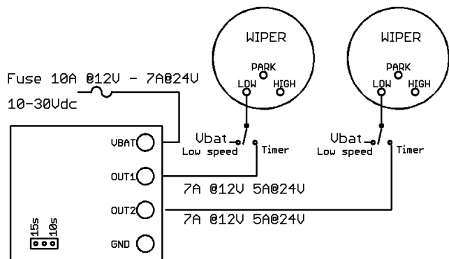
Koblingsskjema
